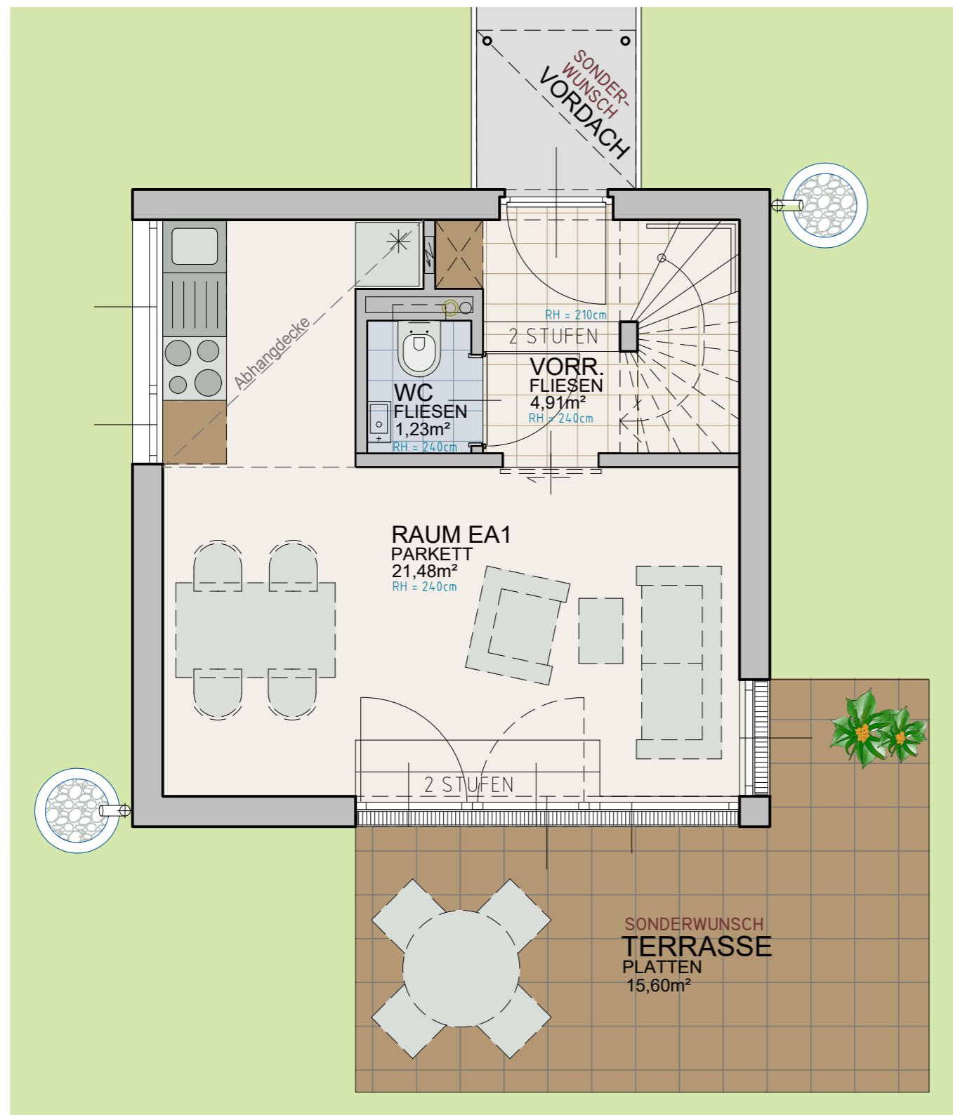
ERDGESCHOSS
